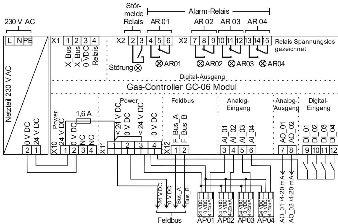
Abbildung 3: GC Modul mit Netzteil
